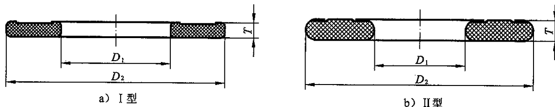
图 4.0.1 垫片的型式
