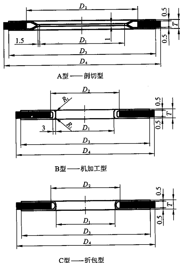
图 3.0.1 垫片的型式
